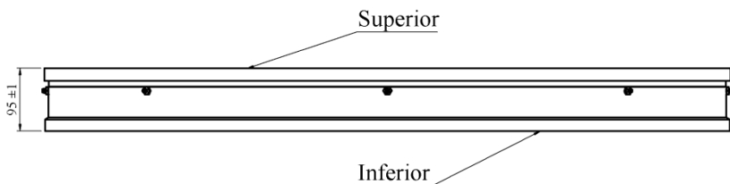
Posição de montagem no equipamento
